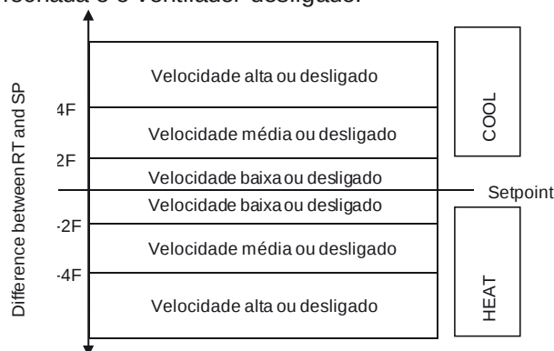
Algoritmo de controle da rampa de velocidade do ventilador
